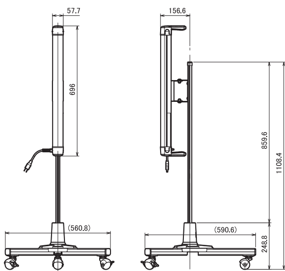
JLS-LED28V、JLS-LED28V-Ra、JLS-LED28V-Rx
