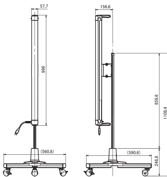
JLS-LED42V、JLS-LED42V-Ra、JLS-LED42V-Rx
