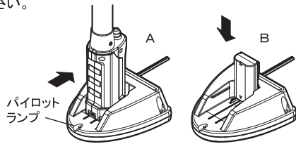
図 4. 充電方法
