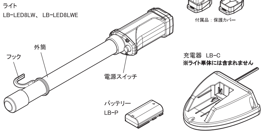
図 1. セット型式（ライト＋充電器＋バッテリー）：LB-LED8W、LB-LED8WE ライト単体型式（ライト＋バッテリー）：LB-LED8LW、LB-LED8LWE
