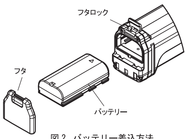
図 2. バッテリー差込方法
