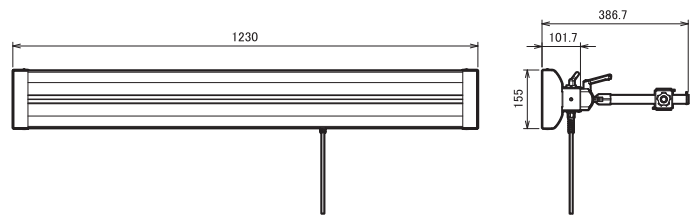
JLS-HF402-A240 照明部
